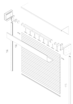
Esploso Sistema Residenziale 400mm; 350mm
