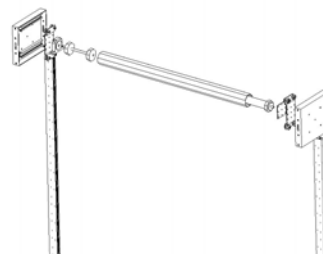
Esploso Sistema Industriale 400mm; 350mm
